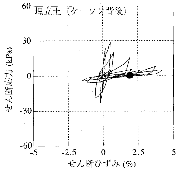
図-8 応力ひずみ曲線 (埋立土)
