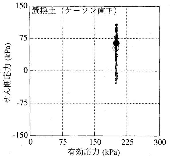
図-20 有効応力経路 (置換土)
