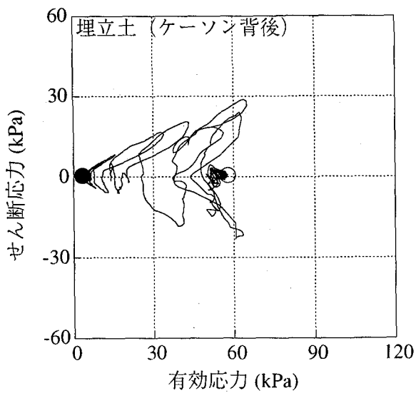
図-7 有効応力経路 (埋立土)
