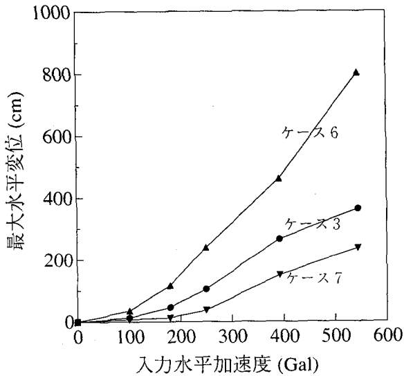
図-13 入力水平加速度と最大水平変位の関係
