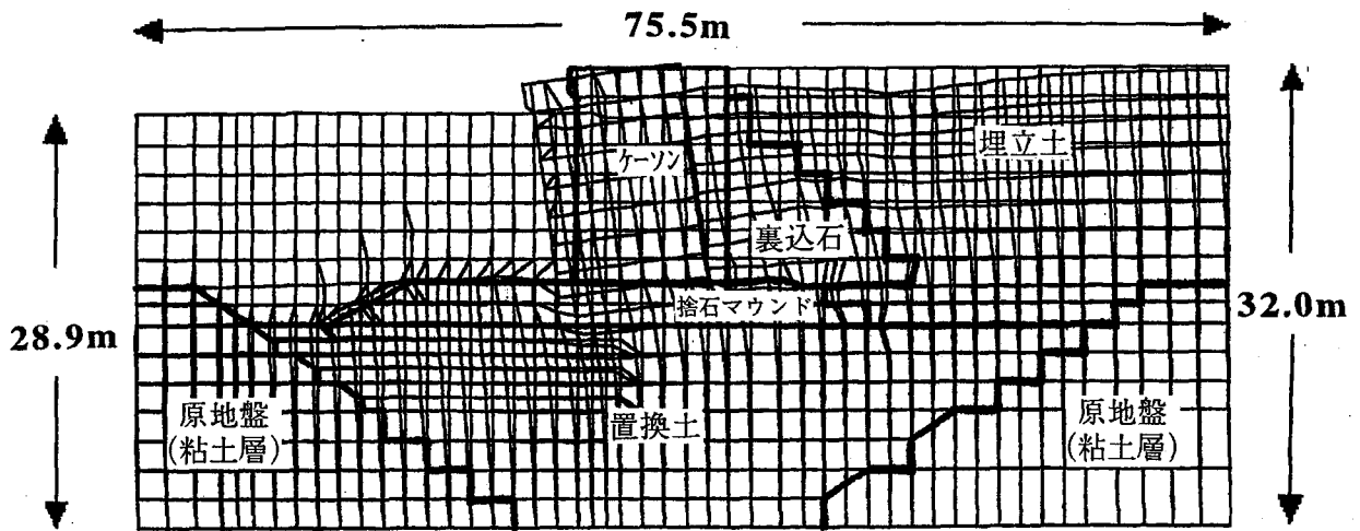
図-6 残留変形図
