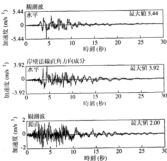
図-3 入力波
