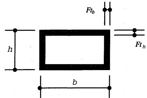
図-2 橋脚断面図
