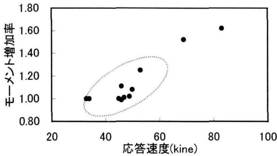
図-12 連結部応答速度と基部モーメント増加率
