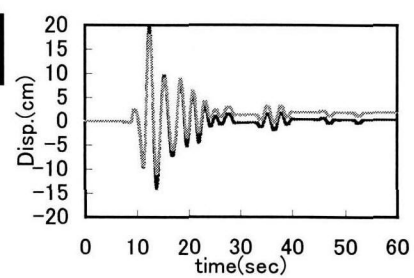
a) G2 桁可動端
