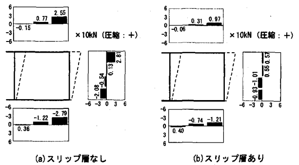
図-18 鉛直方向地盤反力分布 (2径間)
