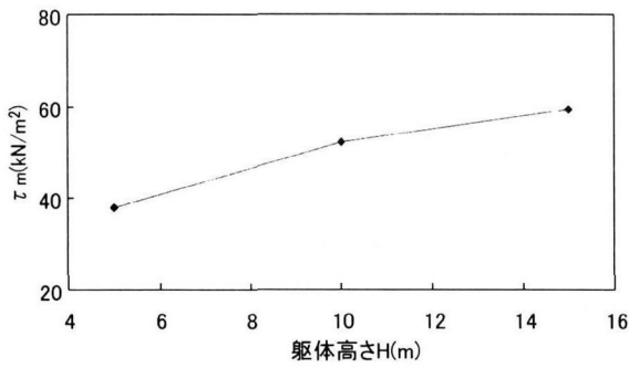
図-7 構造物高さの影響
