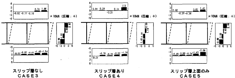
図-20 鉛直方向地盤反力分布 (3径間)
