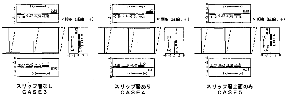
図-19 接線方向地盤反力分布 (3径間)
