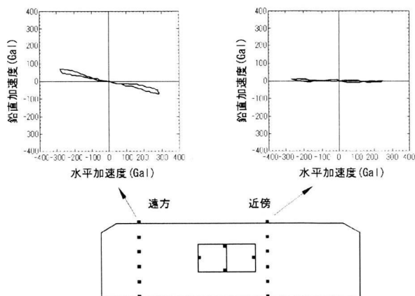
図-16 地盤加速度履歴
