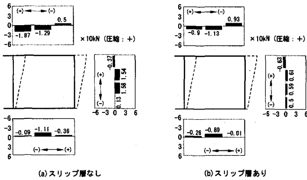
図-17 接線方向地盤反力分布 (2径間)
