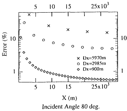
図-3 沖側から入射した場合の屈折誤差 (入射角 80^\circ )
