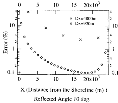
図-4 陸側から反射した場合の屈折誤差 (反射角 10^\circ )
