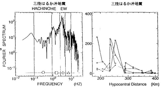
図. 8 FFT法によるフーリエスペクトル
