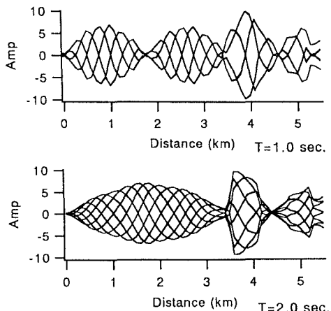
図-4 定常波入射時の変位振幅
