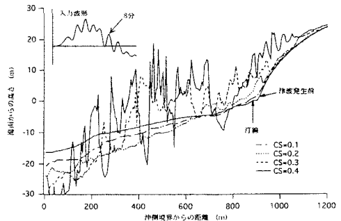
図-4 8分後における地盤高(図-1中の検査断面)
