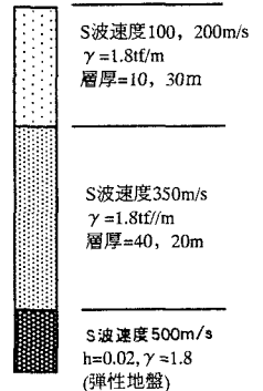
図-1 解析地盤モデル
