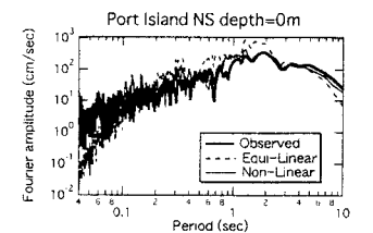
図-5 応答と実測のスペクトル
