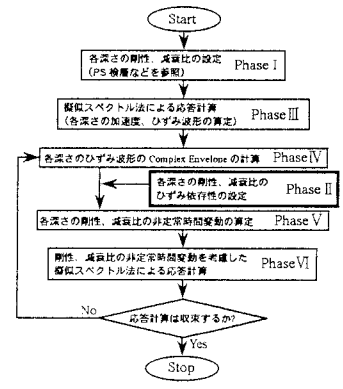
図-1 応答計算のフローチャート
