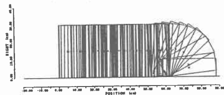
図5(b) 水平軸および鉛直軸を正弦波として入力した場合のシミュレーション結果( \ddot{X} = A \sin \omega t , \ddot{y} = A \sin \omega t ; A=600\text{gal} , f=2.0\text{Hz} )
