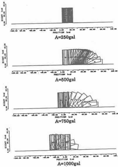
図3 振動数を1.0Hzに固定した場合( \ddot{X} = A \sin \omega t , \ddot{y} = A \sin \omega t ; \omega = 1.01\pi )
