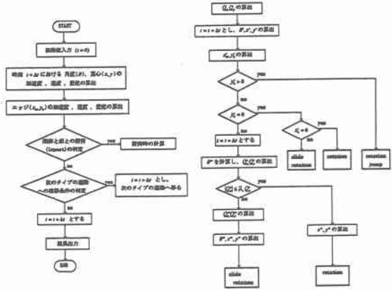
図1 各運動におけるフローチャート 図2 衝突時の計算におけるフローチャート
