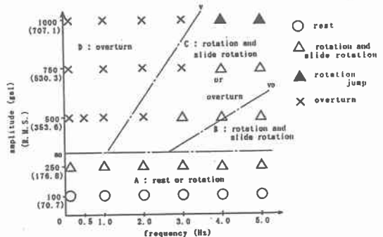
図4 水平軸および鉛直軸を正弦波として入力した場合の剛体の運動 ( \theta \times h = 5 \times 15\text{cm} ; \mu_s = 0.4 , \mu_s = 0.3 ; \epsilon_s = -1.0 , \epsilon_s = 0.0 )
