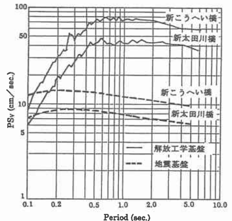
Fig. 2 地震基盤及び解放工学基盤の速度応答スペクトル
