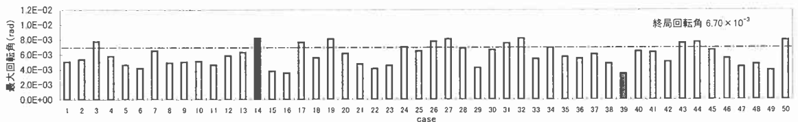
図-3 橋脚基部の塑性ヒンジ部に生じる最大回転角
