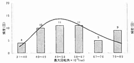
図-4 最大回転角の分布
