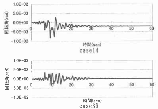
図-7 P2 橋脚の回転角の時刻歴応答波形
