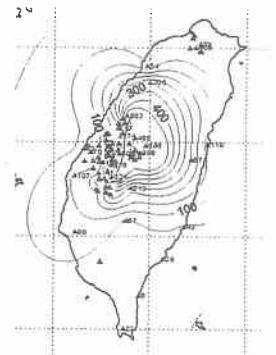
図二 集集地震 最大水平加速度分布 (gal) (東西方向)
