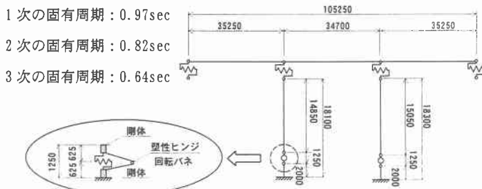
図-3 動的解析モデル 単位：mm
