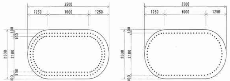
図-2 P2橋脚の断面図 単位：mm
