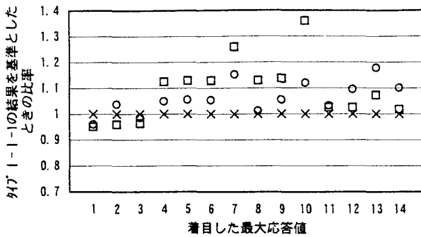
図-11 入力地震動による最大応答値の比較 (タイプI地震動3波)
