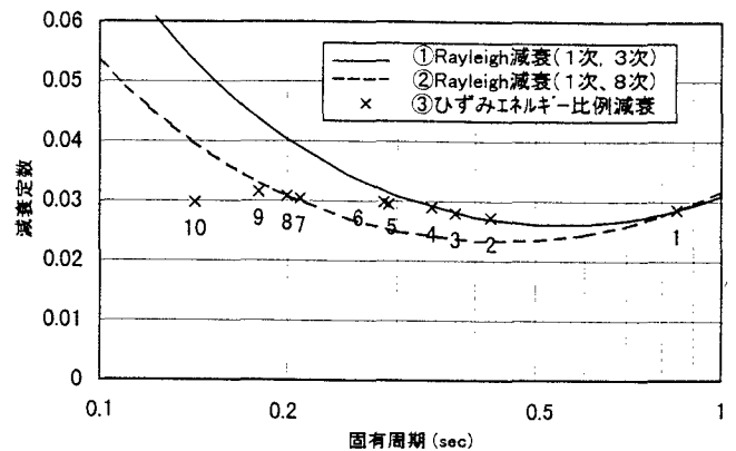
図-9 Rayleigh 減衰とひずみエネルギー比減衰の比較
