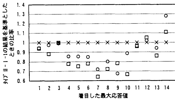
図-12 入力地震動による最大応答値の比較 (タイプII地震動3波)
