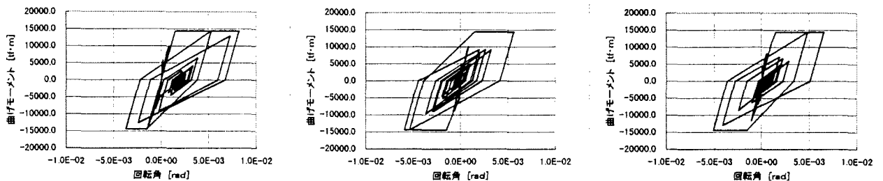
図-13 入力地震動による履歴の比較 (タイプII地震動3波)
