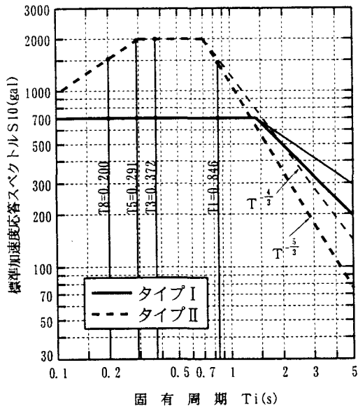
図-3 標準加速度応答スペクトル (I種地盤)
