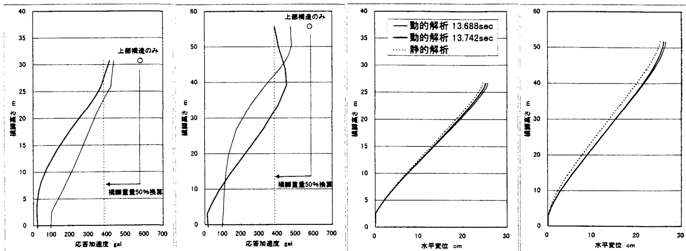
P 1 橋脚
