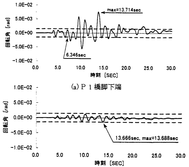
図-4 塑性ヒンジの回転角時刻歴波形 (タイプ I-I-2)
