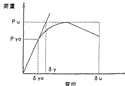
図-5 実験上の降伏変位
