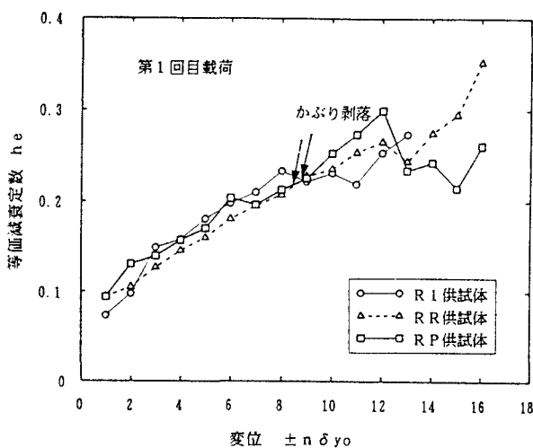
図-7 等価減衰定数
