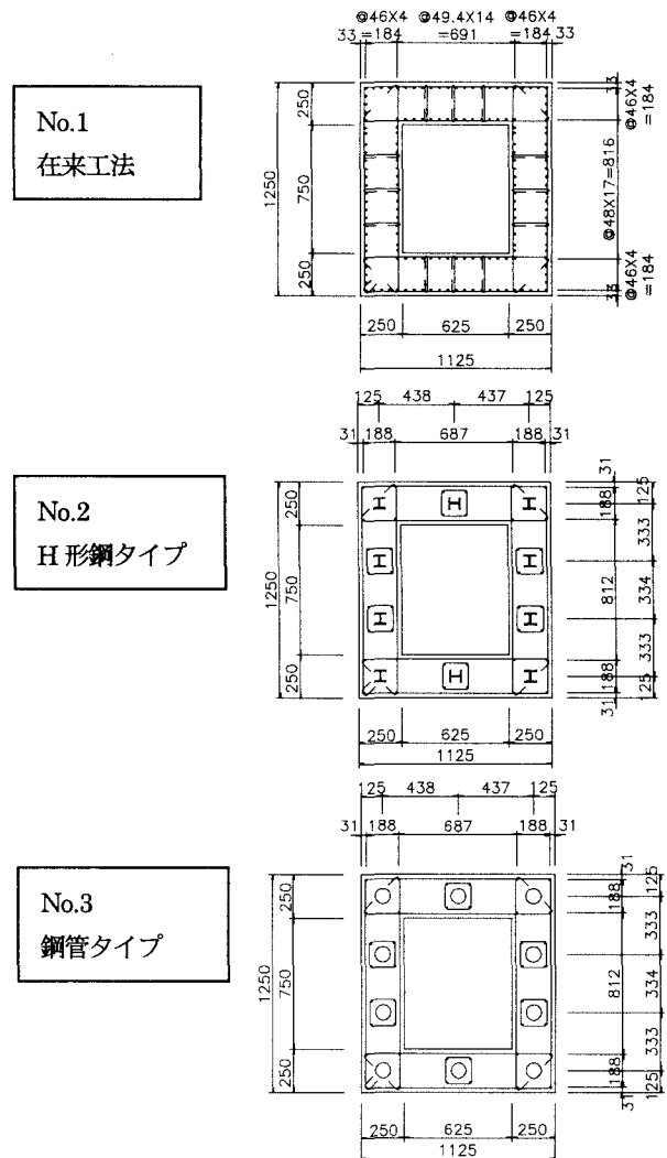
図-2 試験体断面
