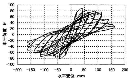
No.3 鋼管タイプ
