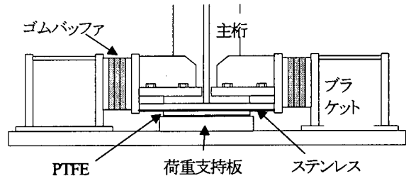
図-2 機能分離型支承装置の取付図
