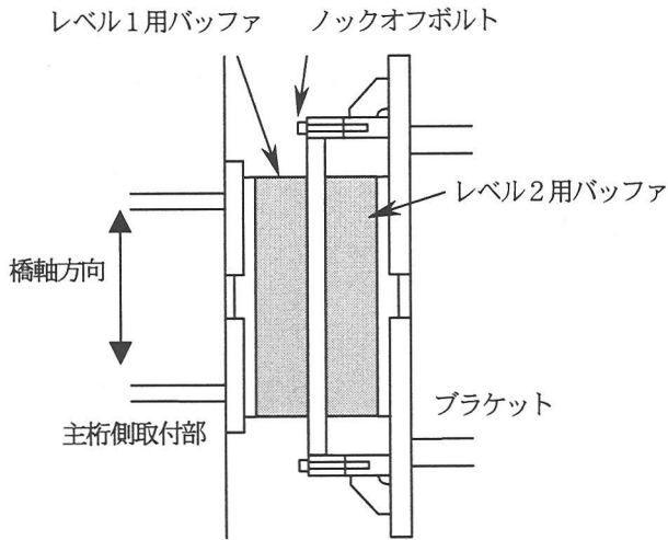
図-3 マルチレベルバッファの平面図
