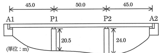
図-4 対象橋梁
