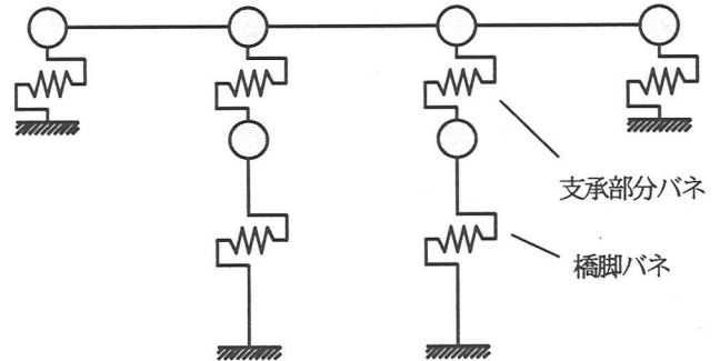
図-5 全体モデル
