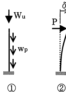
図-7 荷重の載荷方法
