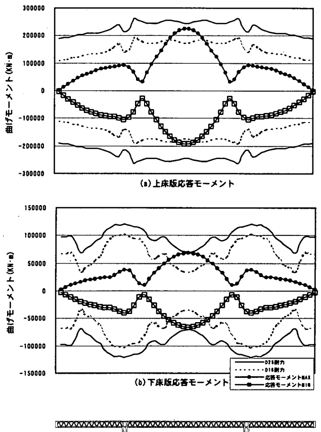
図-8 橋軸直角方向床版照査結果
