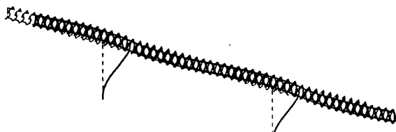
1次モード f=0.749\text{Hz}
