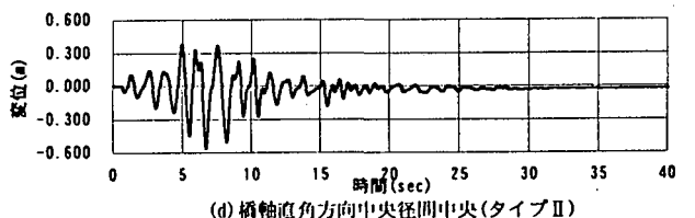
図-5 上部構造の応答変位
