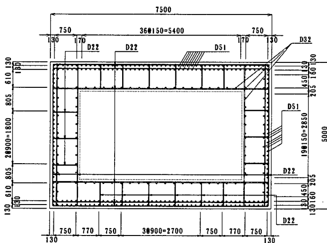
図-3 震度法により決定した鉄筋配置
