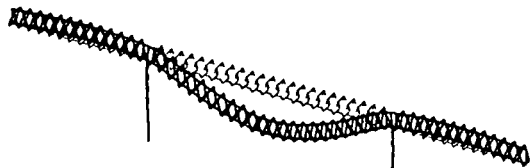
1次モード f=0.749\text{Hz}
