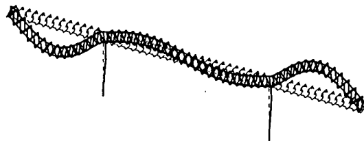
3次モード f=2.551\text{Hz}
