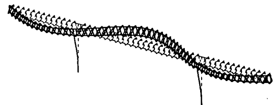
4次モード f=1.982\text{Hz}
