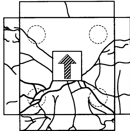
図-3 損傷状況図 (No.1, 3)
