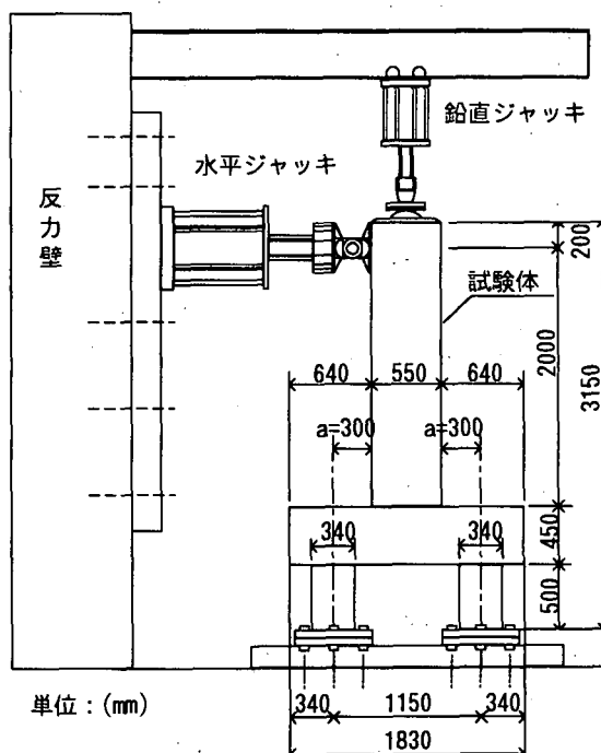
図-1 実験試験体構造図
