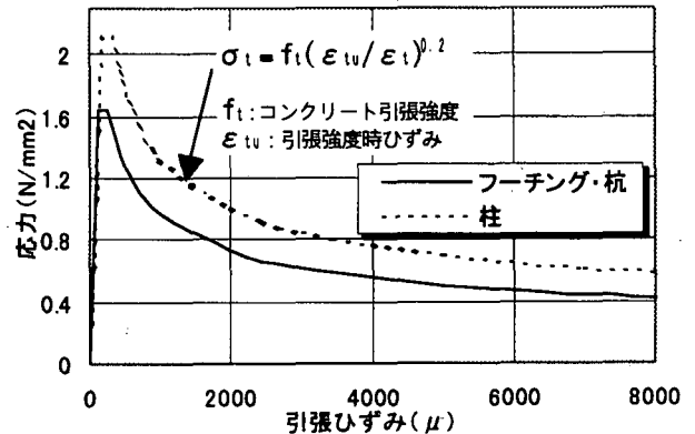
図-7 コンクリートの引張軟化モデル
