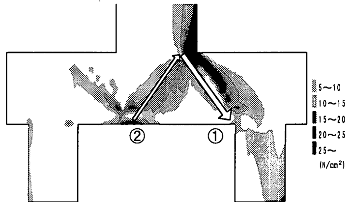
図-17 最大荷重付近での最小主応力分布図 (No.2 試験体)
