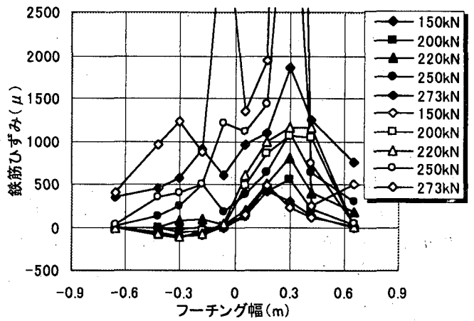
図-13 フーチング下面鉄筋ひずみ分布
