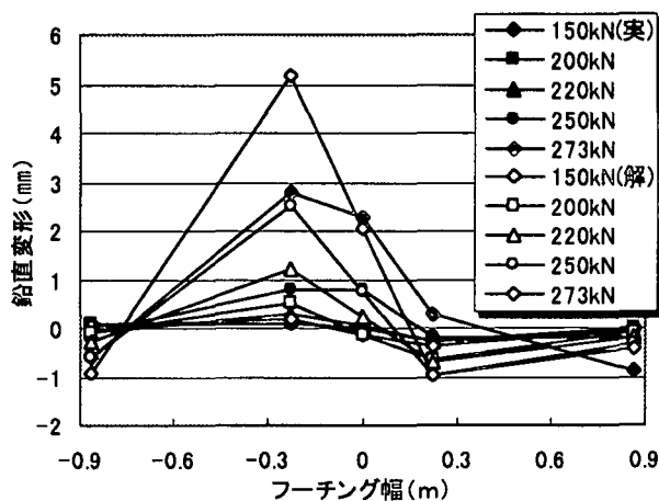
図-9 フーチングの鉛直変形-荷重の関係
