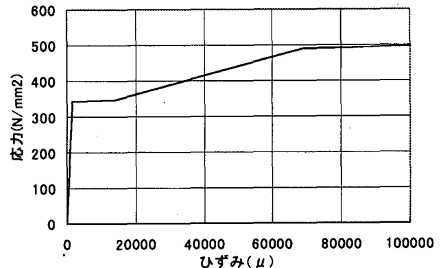
図-8 鉄筋の応力-ひずみモデル
