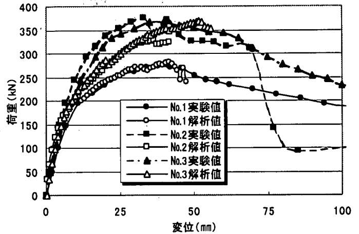
図-2 各試験体の柱天端の水平変位-荷重の関係
