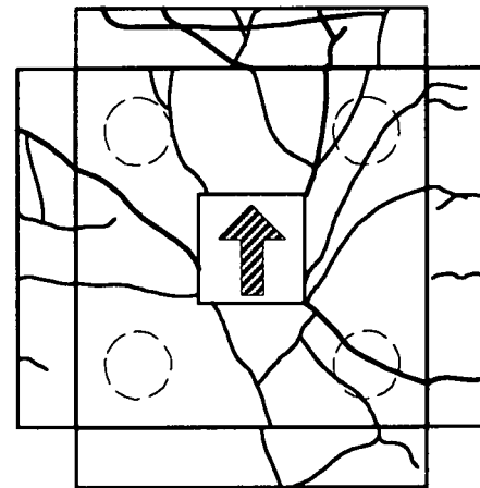
図-4 損傷状況図 (No.2)
