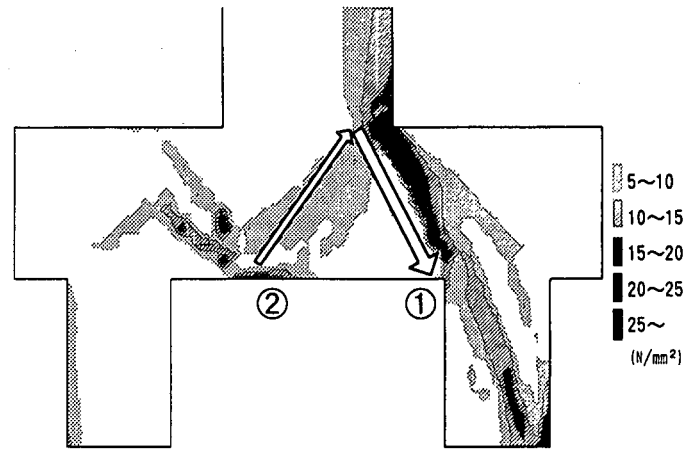
図-16 最大荷重付近での最小主応力分布図 (No.1 試験体)
