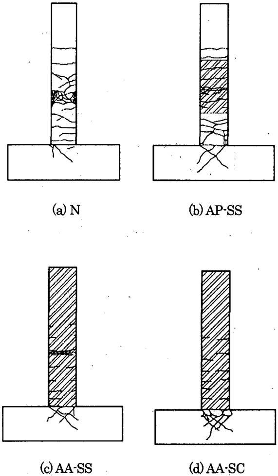
図-5 試験体破壊性状
