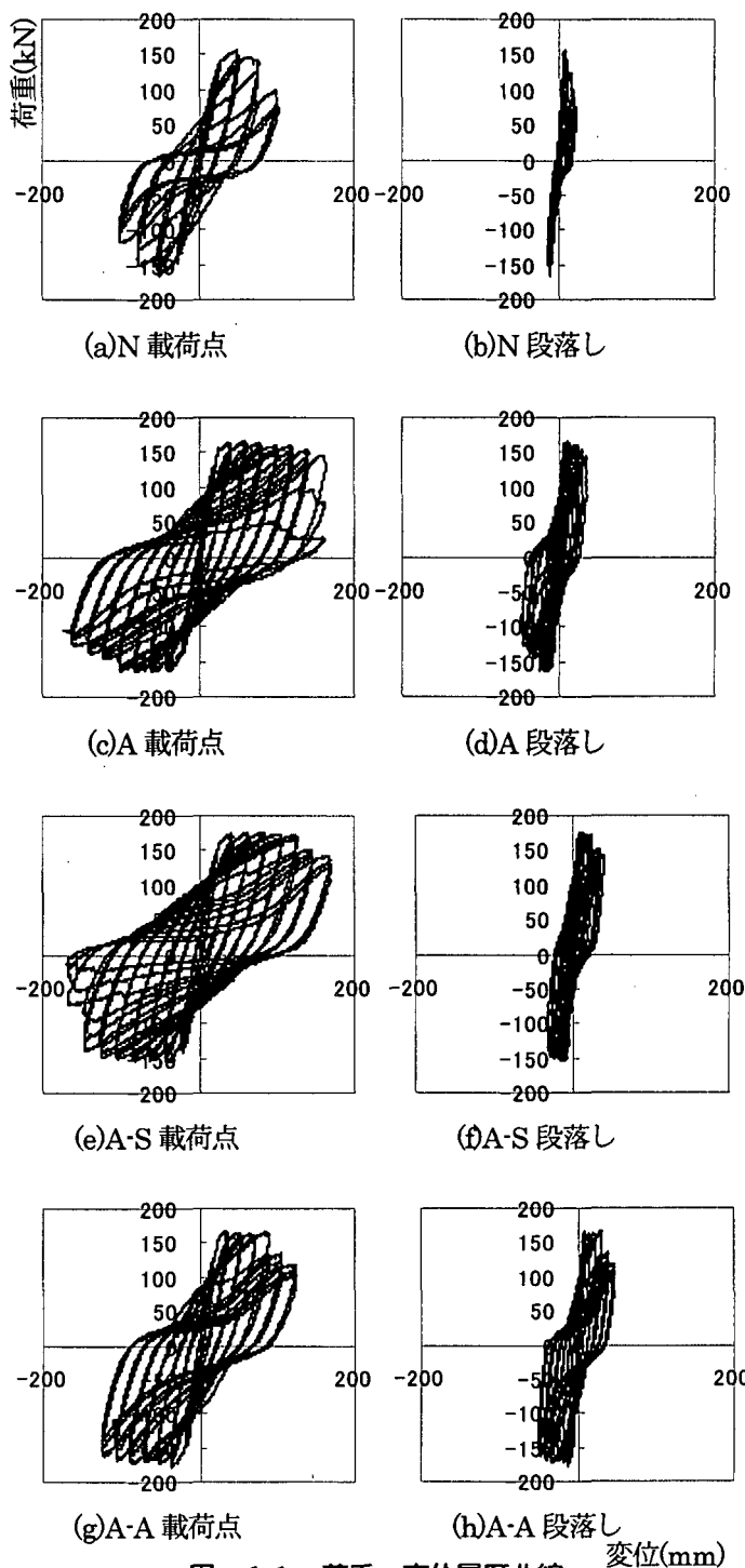
図-11 荷重-変位履歴曲線
