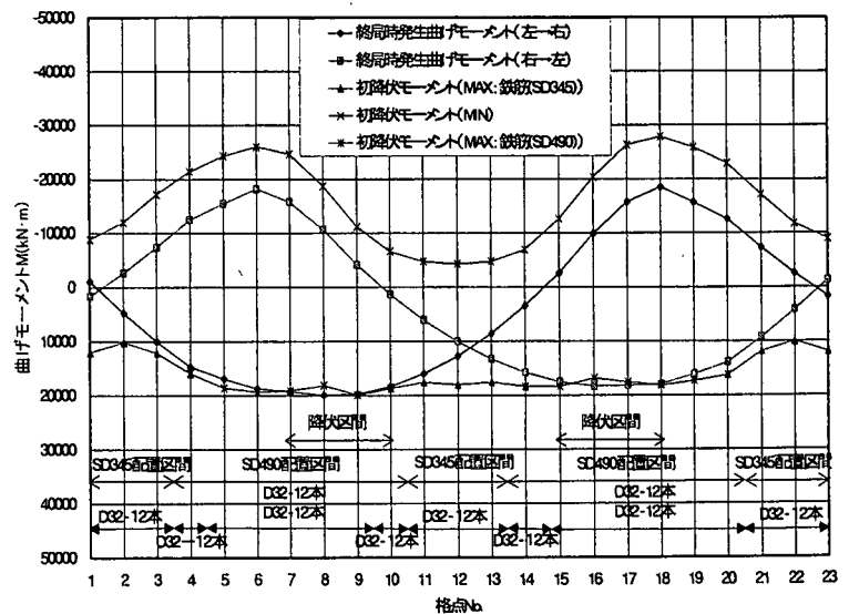
図-8 B(1)案 発生曲げモーメント図(SD490案)
