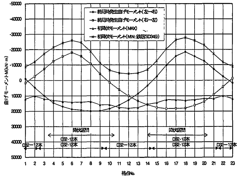
図-4 発生曲げモーメント図（鉄筋案）
