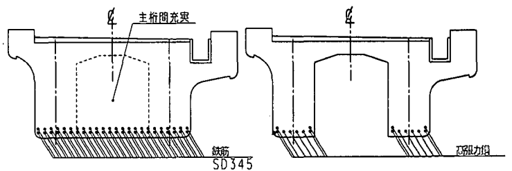
A) 主桁断面拡大案 B) 鉄筋代替案
