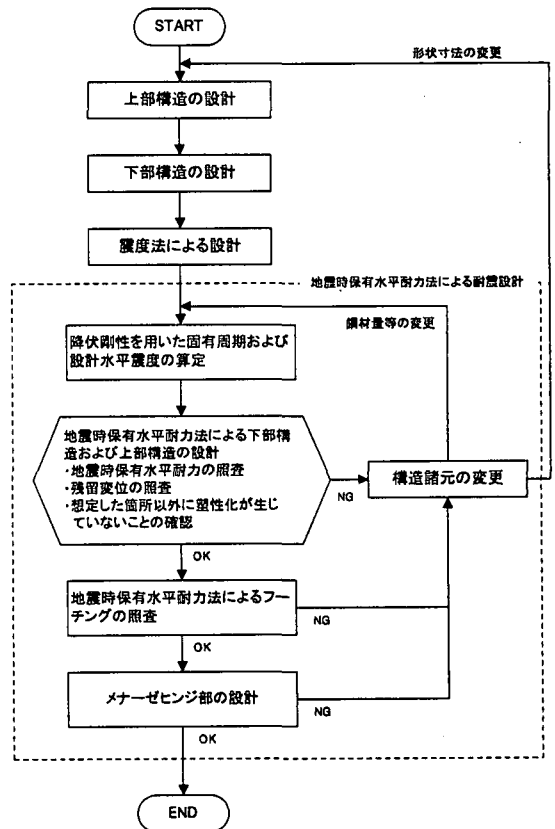
図-1 斜 \pi 橋の設計計算の流れ
