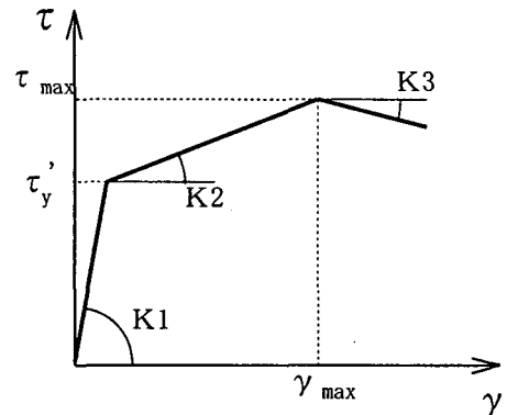
図-10 せん断応力-せん断ひずみ関係
