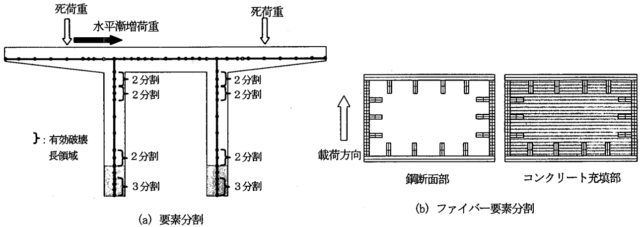
図-2 解析モデル (梁部弾性挙動)
