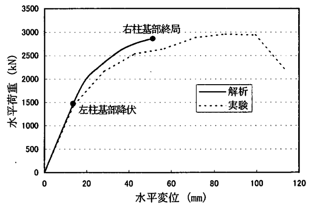
図-4 解析結果と実験結果の比較
