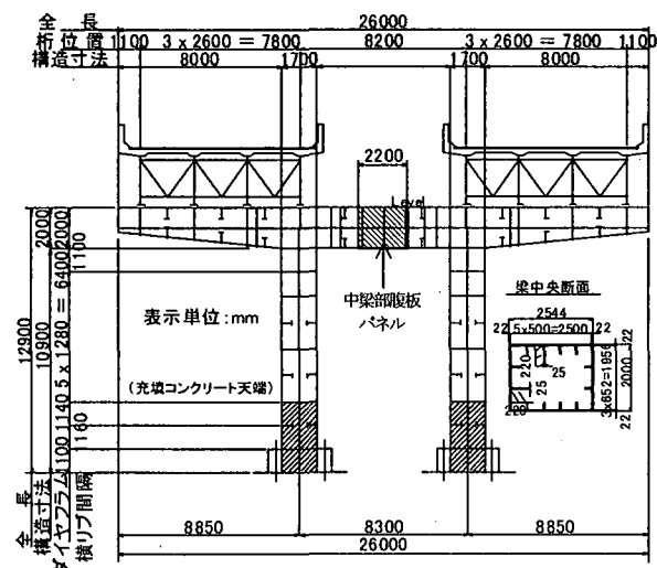
図-1 対象ラーメン橋脚
