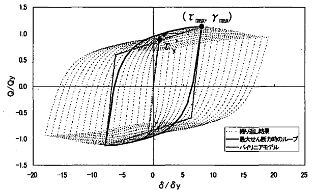
図-11 パラメータ (\tau_y', K2) の算出
