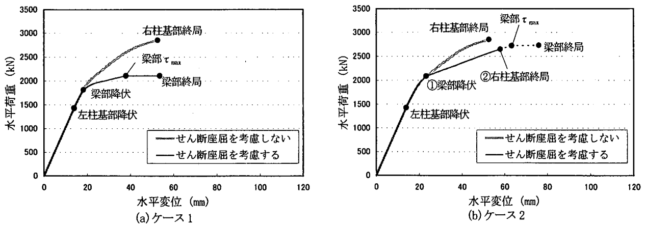
図-8 梁実験スケルトンを組み込んだ解析
