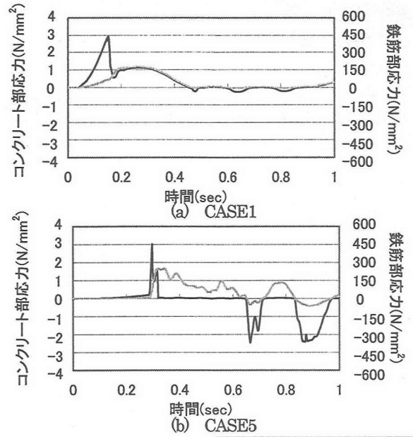
図-15 橋台基部の曲げ応力値の比較
