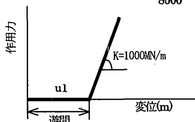
図-4 衝突バネモデル
