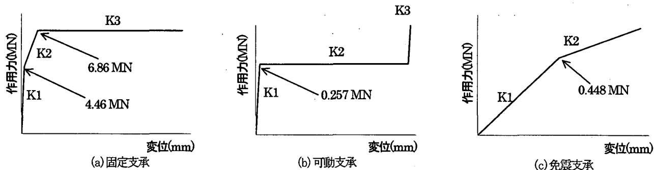
図-6 支承モデル
