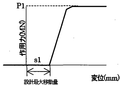
図-10 落橋防止バネモデル
