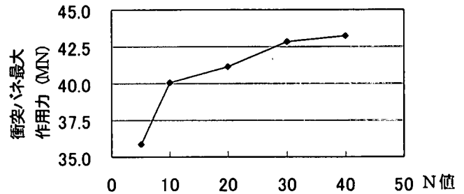
図-9 背面地盤の違いによる 衝突パネ最大作用力の影響
