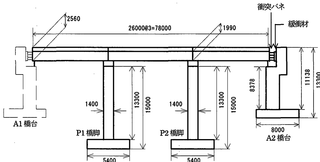
図-11 連続桁橋解析モデル図
