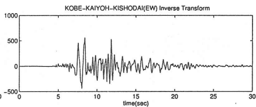
図3 ウェーブレット変換結果を逆変換して得られた再構成波形
