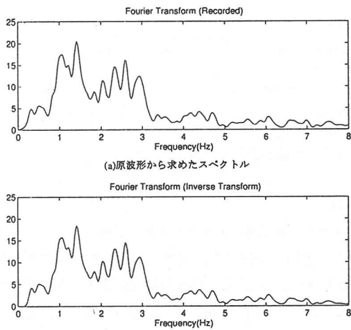
図4 原波形・再構成波形のフーリエスペクトル
