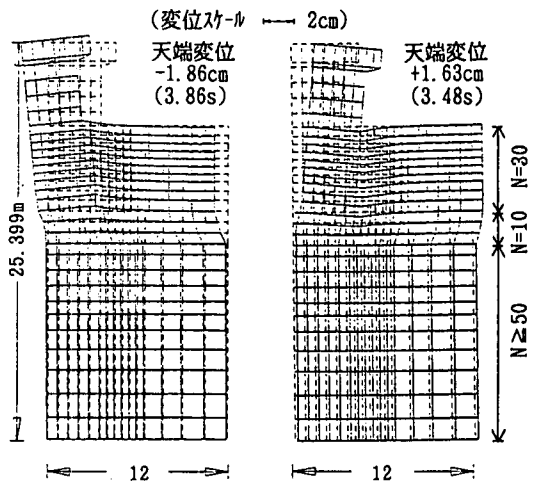
図9 変形図 (Model-1R)
