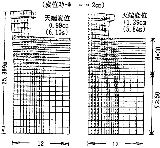
図8 変形図 (Model-1N)
