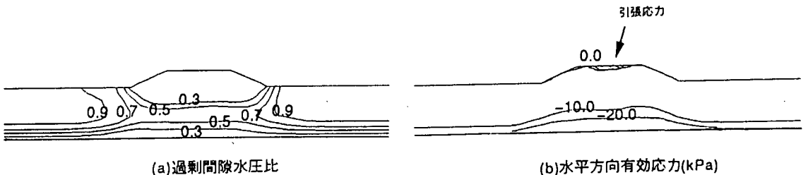
図-4 過剰間隙水圧比と水平方向有効応力の分布(ケース1, t=1.5秒)
