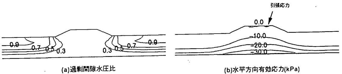
図-10 過剰間隙水圧比と水平方向有効応力の分布 (ケース4, t=4 秒)
