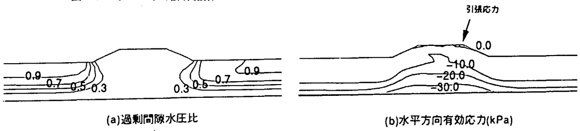
図-8 過剰間隙水圧比と水平方向有効応力の分布 (ケース3, t=4 秒)
