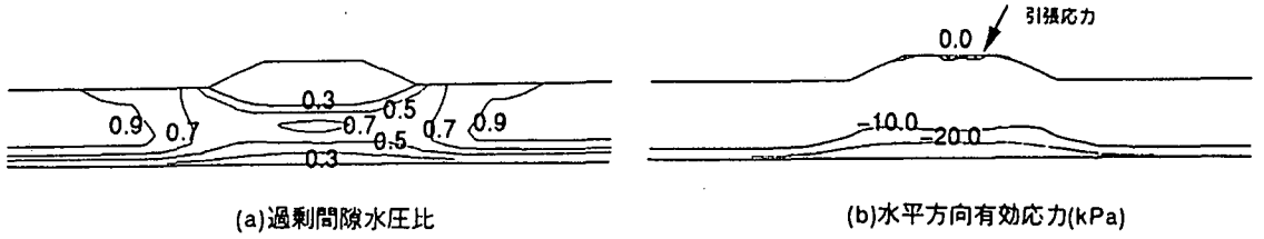
図-6 過剰間隙水圧比と水平方向有効応力の分布 (ケース2, t=1.5 秒)
