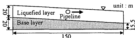
図10 実スケール地盤モデル
