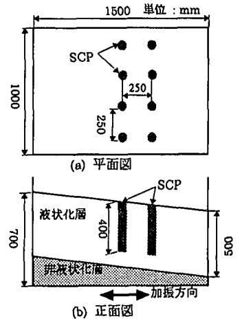
図4 模型実験の概要図
