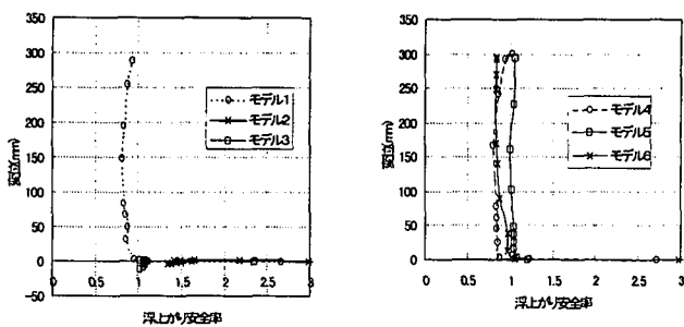
図-7 浮上がり変位と安全率の関係
