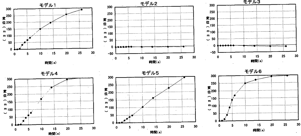
図-3 浮上り変位の時刻歴
