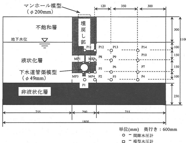
図-1 模型概要
