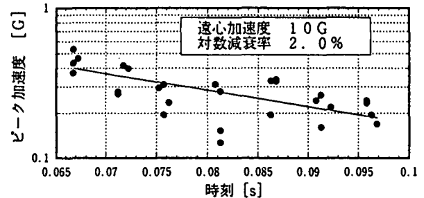
図-10 消波工堤体の対数減衰率
