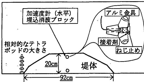
図-8 消波工堤体概要
