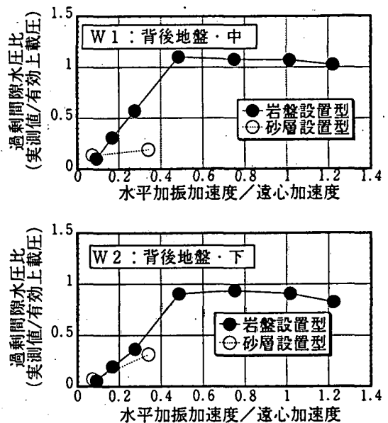
図-6 入力加速度-過剰間隙水圧比関係
