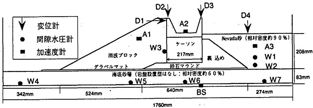
図-1 模型断面図
