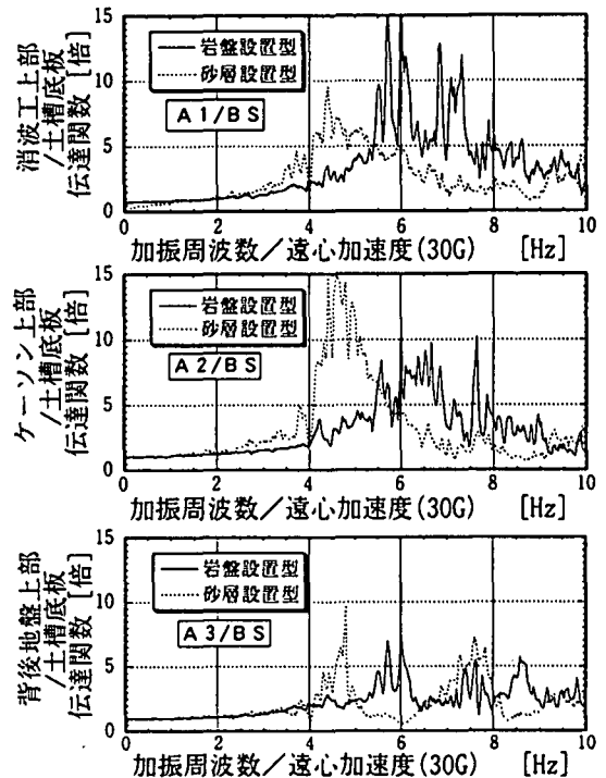
図-4 模型各部の伝達関数
