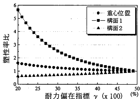
図-4. 塑性率比と偏在指標の関係
