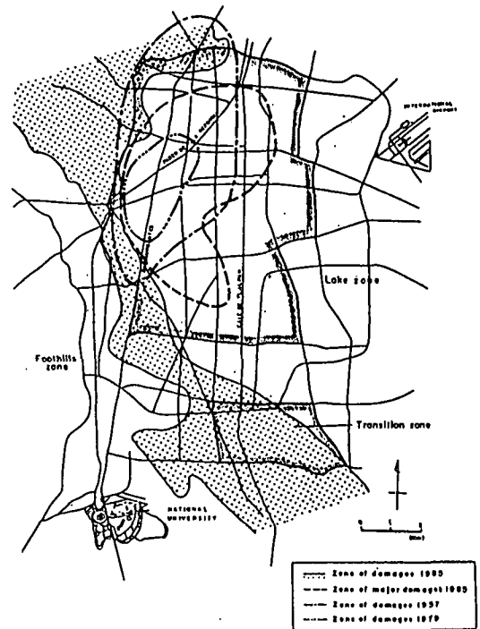
図-11 過去の地震によるメキシコシティ被害域
