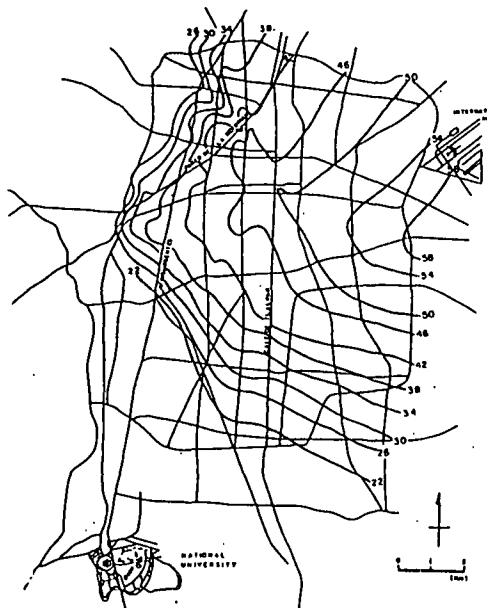
図-10 メキシコシティ超軟弱層コンター
