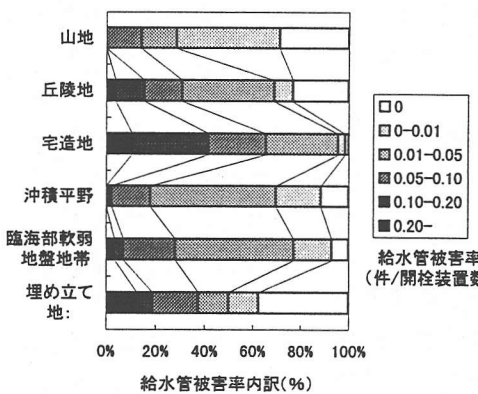
図4 代表地形による配水管・給水管被害率
