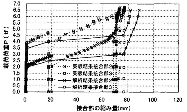
図-12 接合部の縮み量
