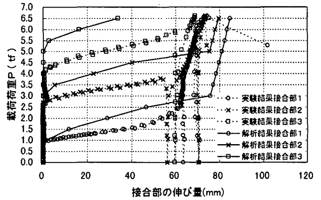
図-10 接合部の伸び量
