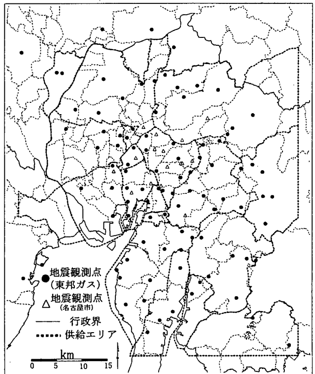
図-1 名古屋地域の地震計配置図
