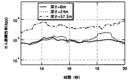
図-15 各深さのせん断剛性の時間変動の比較 (余震 1, EW 成分)
