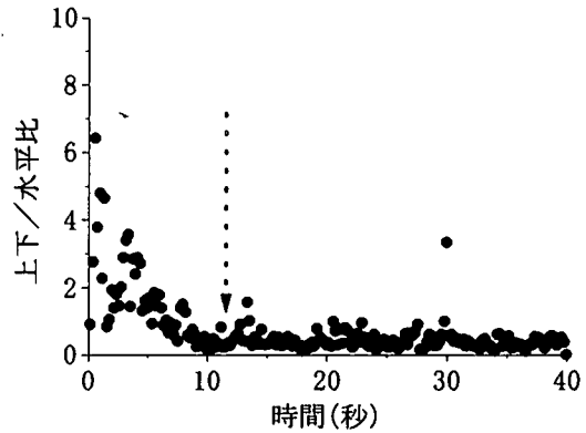
図-2 森河内の上下/水平比 (時間間隔 \delta_t: 0.2 秒)
