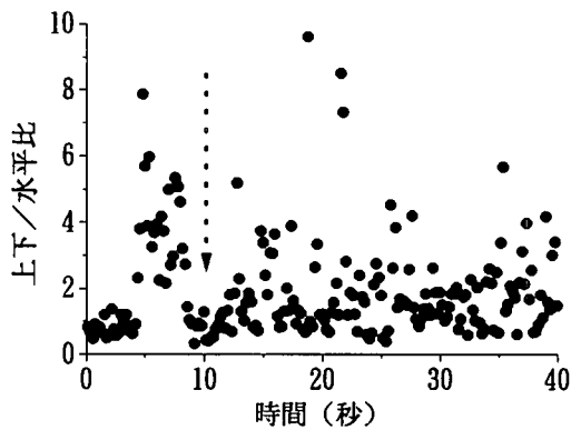
図-1 ポートアイランドの上下/水平比 (時間間隔 \delta_t: 0.2 秒)
