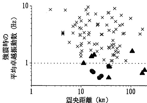
図-5 強震時の平均卓越振動数と震央距離の関係
