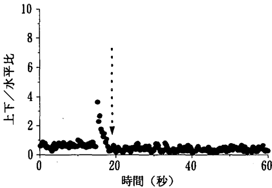
図-3 阿久根の強震記録の上下/水平比 (地震: EQ. 1)
