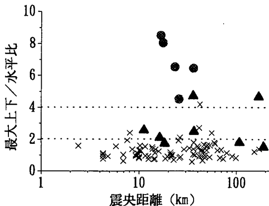
図-4 最大上下/水平比と震央距離の関係
