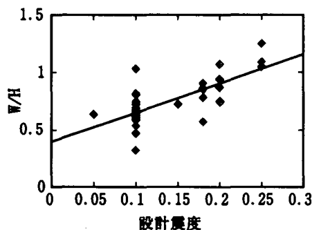
図-2 設計震度とW/Hの関係
