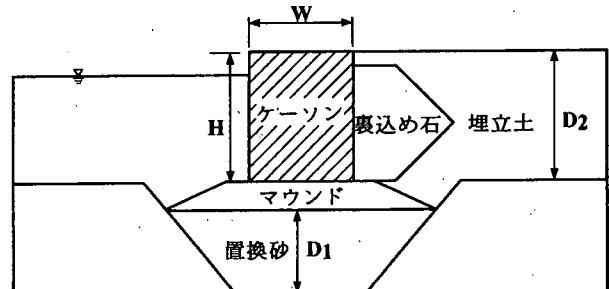
図-1 重力式岸壁の標準断面図
