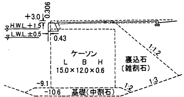
(a) 釧路港第二埠頭地区西側岸壁(-9.0m)
