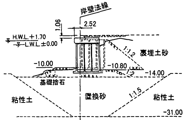
(b) 神戸港六甲アイランド-10m岸壁 (Tバース)
