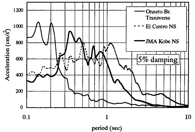
図7 各地震波の絶対加速度応答スペクトル
