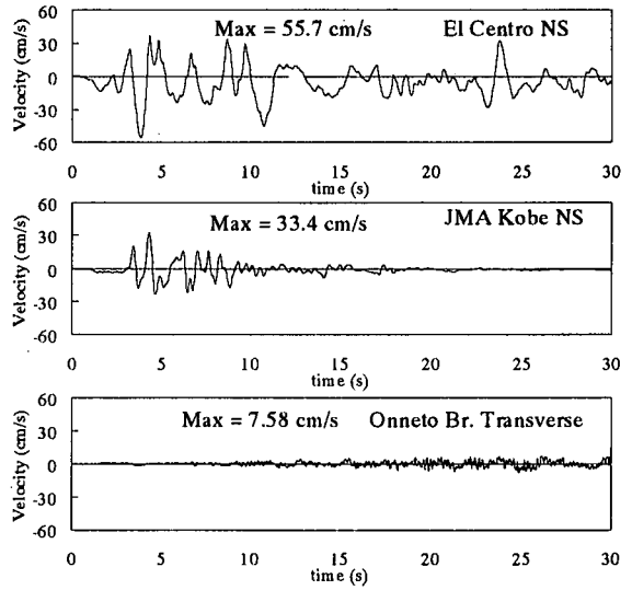
図6 各地震波の水平方向の速度波形
