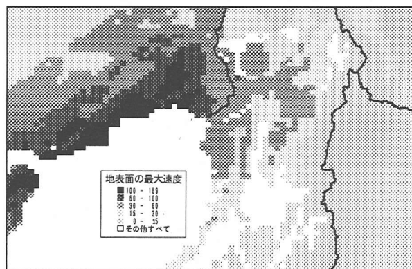
図 2 兵庫県南部地震の地表面最大速度の推定分布
