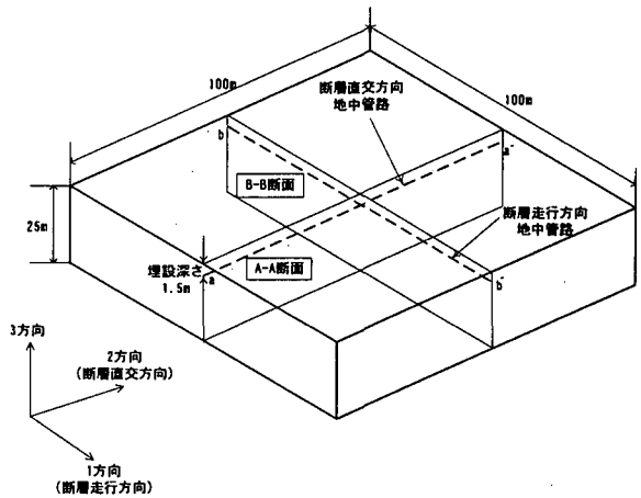
図5 3次元地盤モデル図の概要
