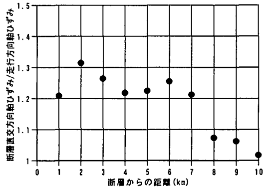
図 9 断層からの距離と軸方向ひずみの比
