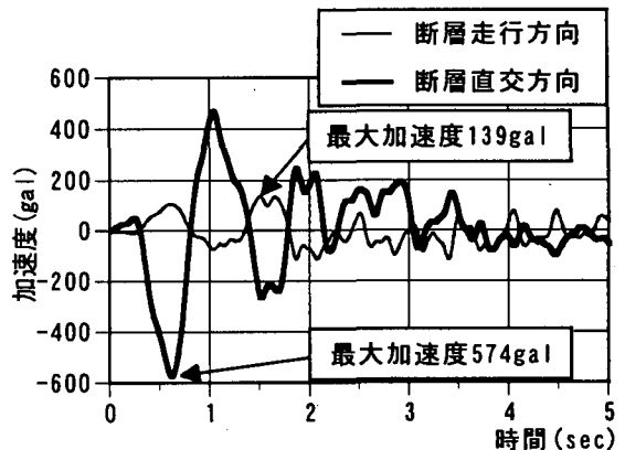
図6 入力地震動の一例(断層からの距離2km)
