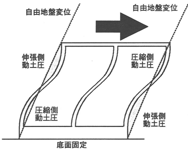
図-1 変形が小さい場合の動土圧の分布
