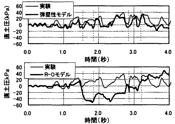
図-8 側壁に作用する動土圧時刻歴の比較
