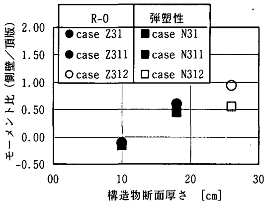
図-10 断面厚さとモーメント比の関係
