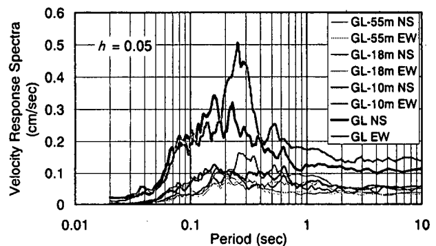
図-7 地盤の速度応答スペクトル
