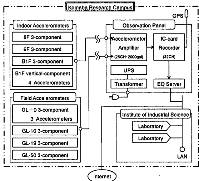
図-5 地震観測システムの構成
