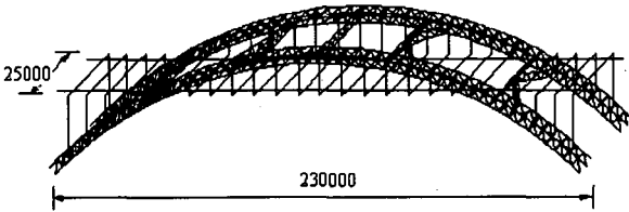
図-2 解析対象橋の一般図 (単位: mm)
