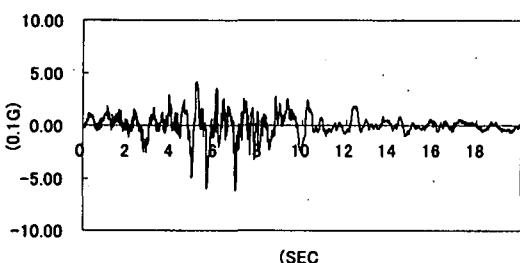
(b) 東神戸大橋観測波 (Case11~Case13) 図-2 入力地震動
