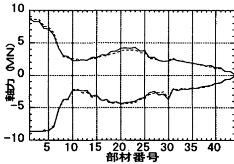
(a) 補剛桁の最大軸力
