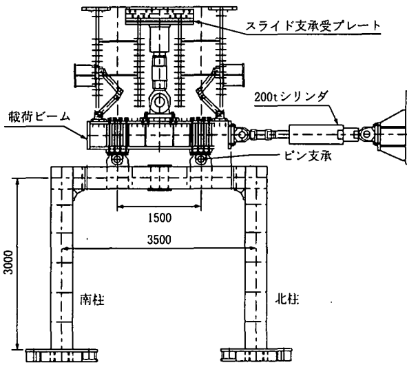
図-1 供試体および荷装置の概略図
