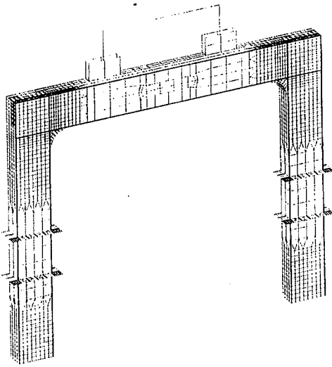
図-3 FEM解析モデル
