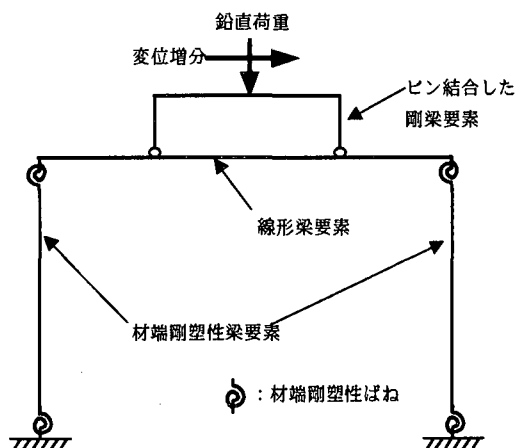
図-9 簡易解析モデル
