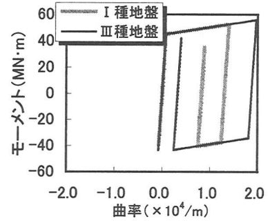
図-11 P2 橋脚基部の曲率-曲げモーメント
