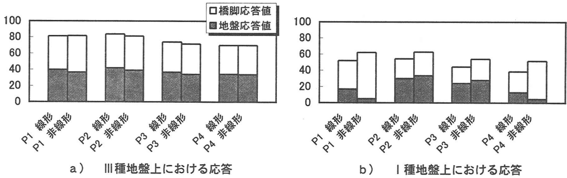
図-9 橋脚天端における変位置 (スパン長 200m)
