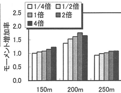
図-17 衝突バネ剛性がモーメント増加率に及ぼす影響
