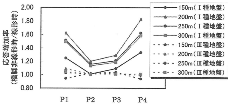
図-10 橋脚天端における応答変位増加率
