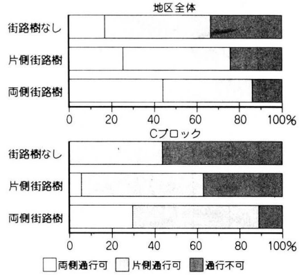
図-13 街路樹の有無別に見た歩道通行可否状況
