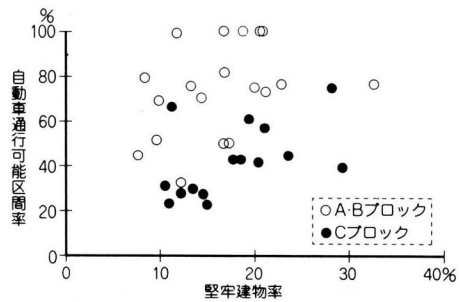
図-14 堅牢建物の割合と道路被害状況
