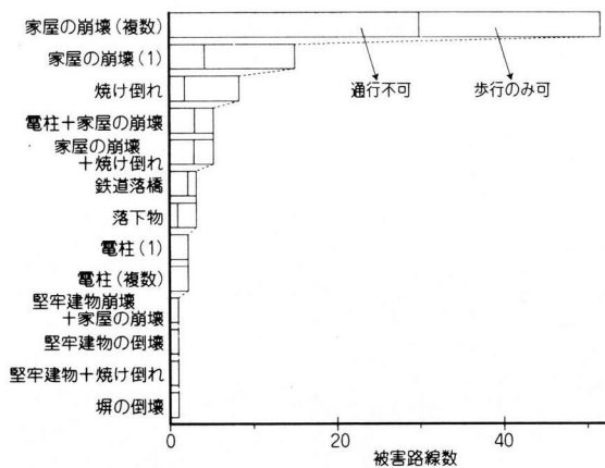
図-7 道路の閉塞原因
