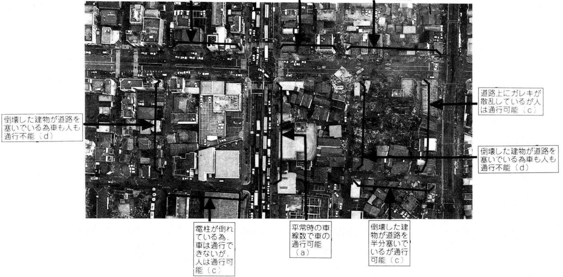
図-1 道路閉塞状況の判読事例
