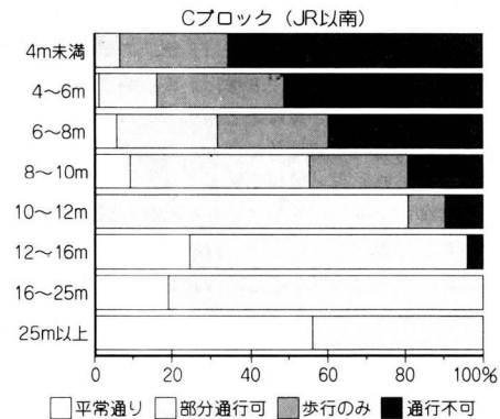
図-10 ブロック別・幅員別にみた道路被害状況
