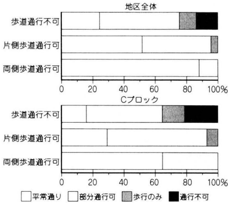
図-12 歩道の通行可否別に見た道路被害状況
