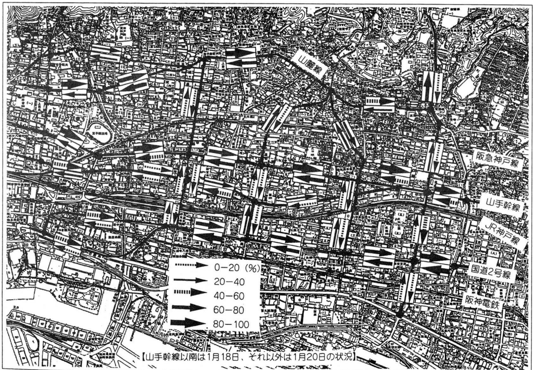
図-5 補助幹線道路を含めた主要な道路における走行車両率
