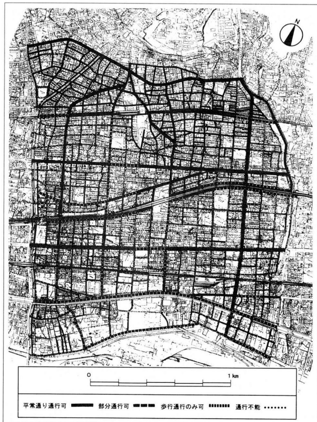
図-6 道路被害状況
