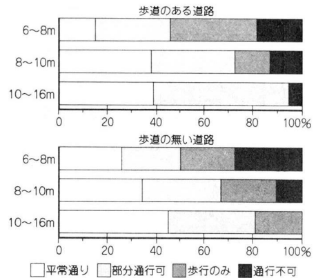
図-11 歩道の有無別にみた道路被害状況
