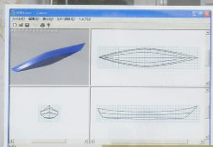
カヌー設計ソフト
